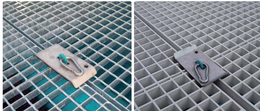
Kluitenrooster in gegalvaniseerd staal of polyester (optioneel)
