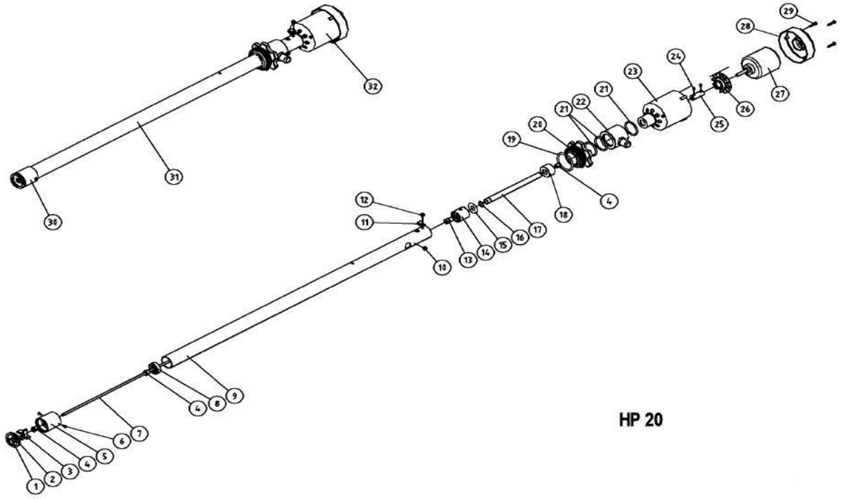
Varaosakuva nro 11 Partspicture No 11 Pumppu Pump
