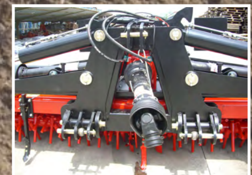
Tripuntal frontal con bulón pivotante Atelage frontal avec boulon pivotant Pivoting rod coupling set
